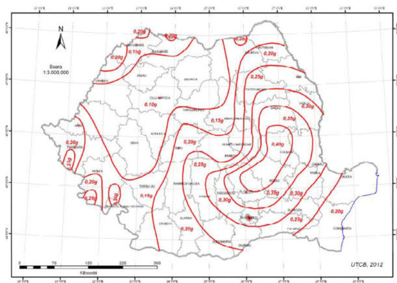
Zonarea teritoriului României în termeni de valuri de accelerații terenului pentru proiectare ag pentru cutremure având intervalul mediu de recurență IMR = 225 ani și 20% posibilitate de depășire în 50 de ani.
