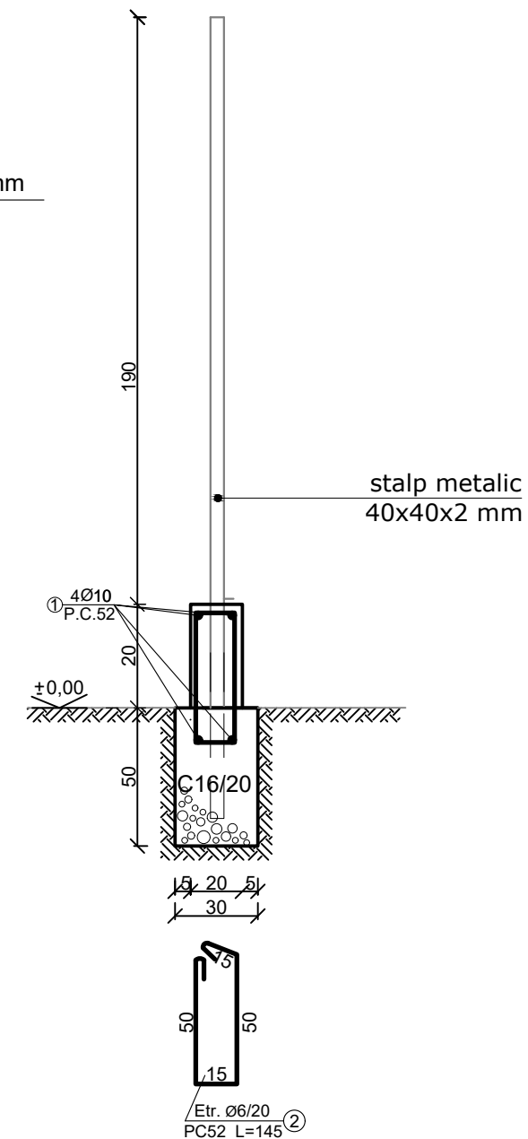
Sectiunea1-1 prin imprejmuire din plasa metalica bordurata h=2.10 m scara 1:20
