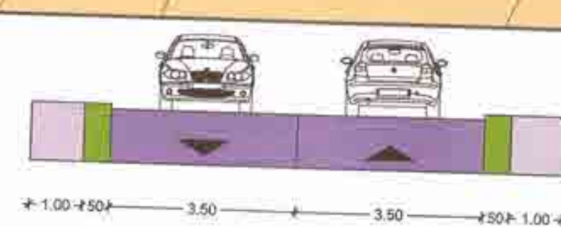
SECTIUNE C-C' - Str. Miraslau scara 1:100
