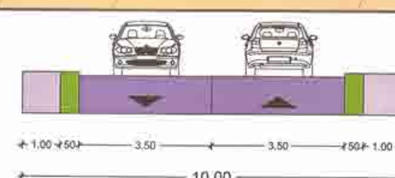
SECTIUNE C-C' - Str. Miraslau scara 1:100
