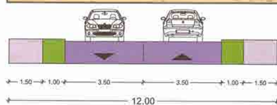
SECTIUNE A-A' - Str. Biruintei scara 1:100
