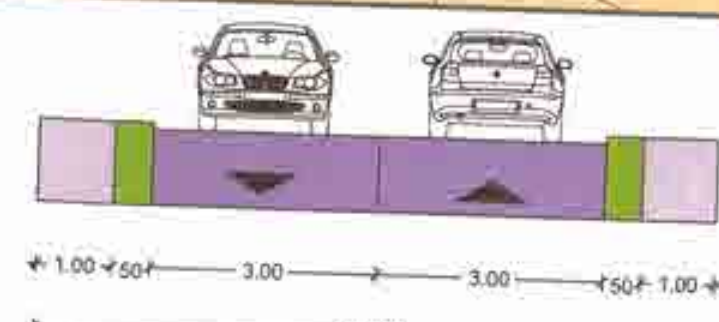
SECTIUNE B-B' - Cale de acces scara 1:100
