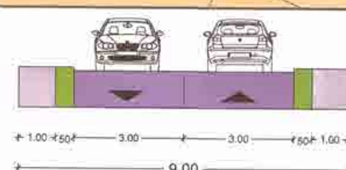
SECTIUNE B-B' - Cale de acces scara 1:100
