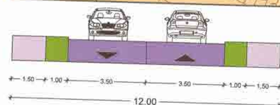
SECTIUNE A-A' - Str. Biruintei scara 1:100
