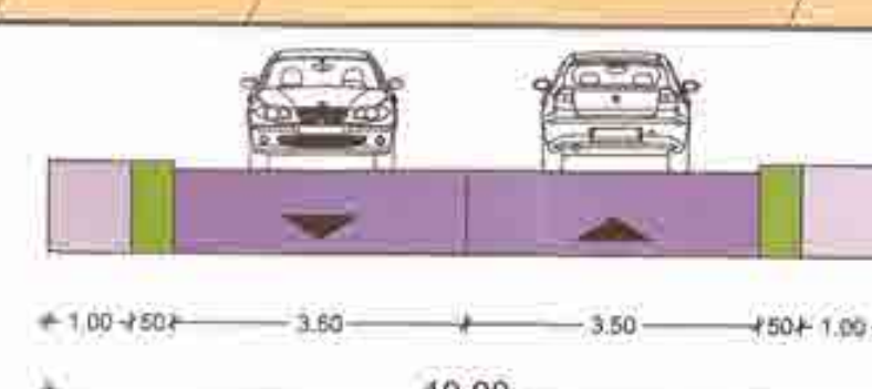
SECTIUNE C-C' - Str. Miraslaui scara 1:100
